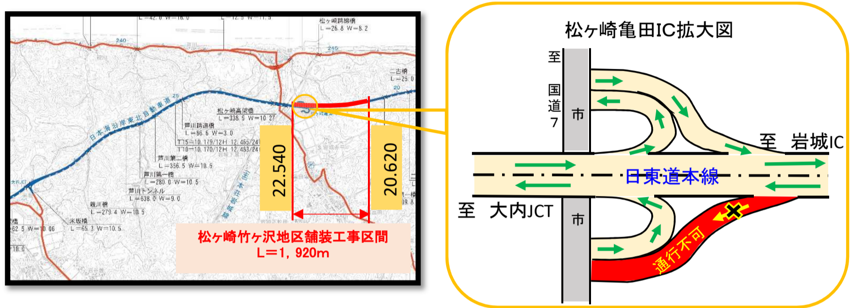
◎車線切り替え後平面図
