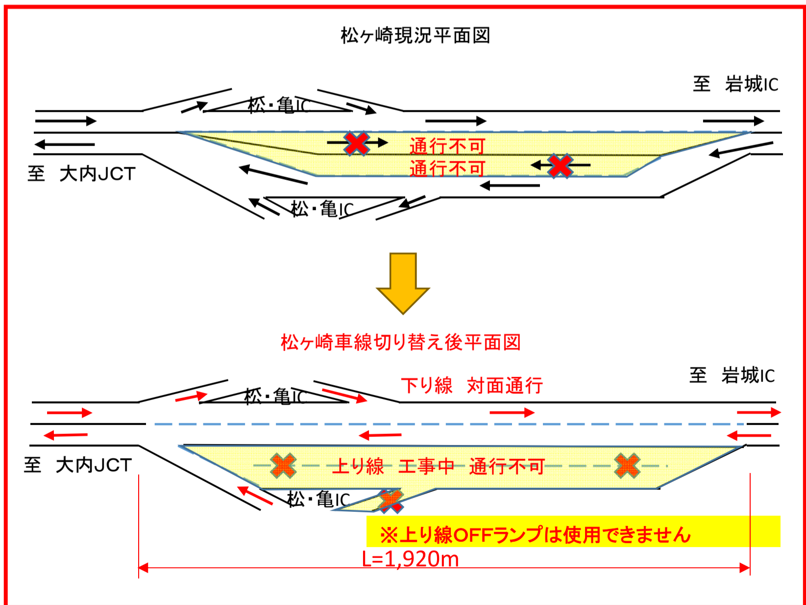
◎車線切り替え後平面図
